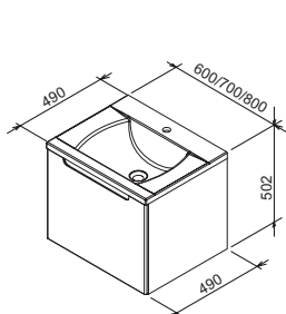
SD Classic 600/700/800-L/R
