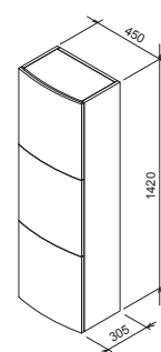
SB Evolution uzavřený
