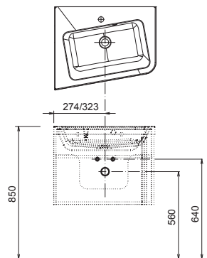
SD 10° rohová L
